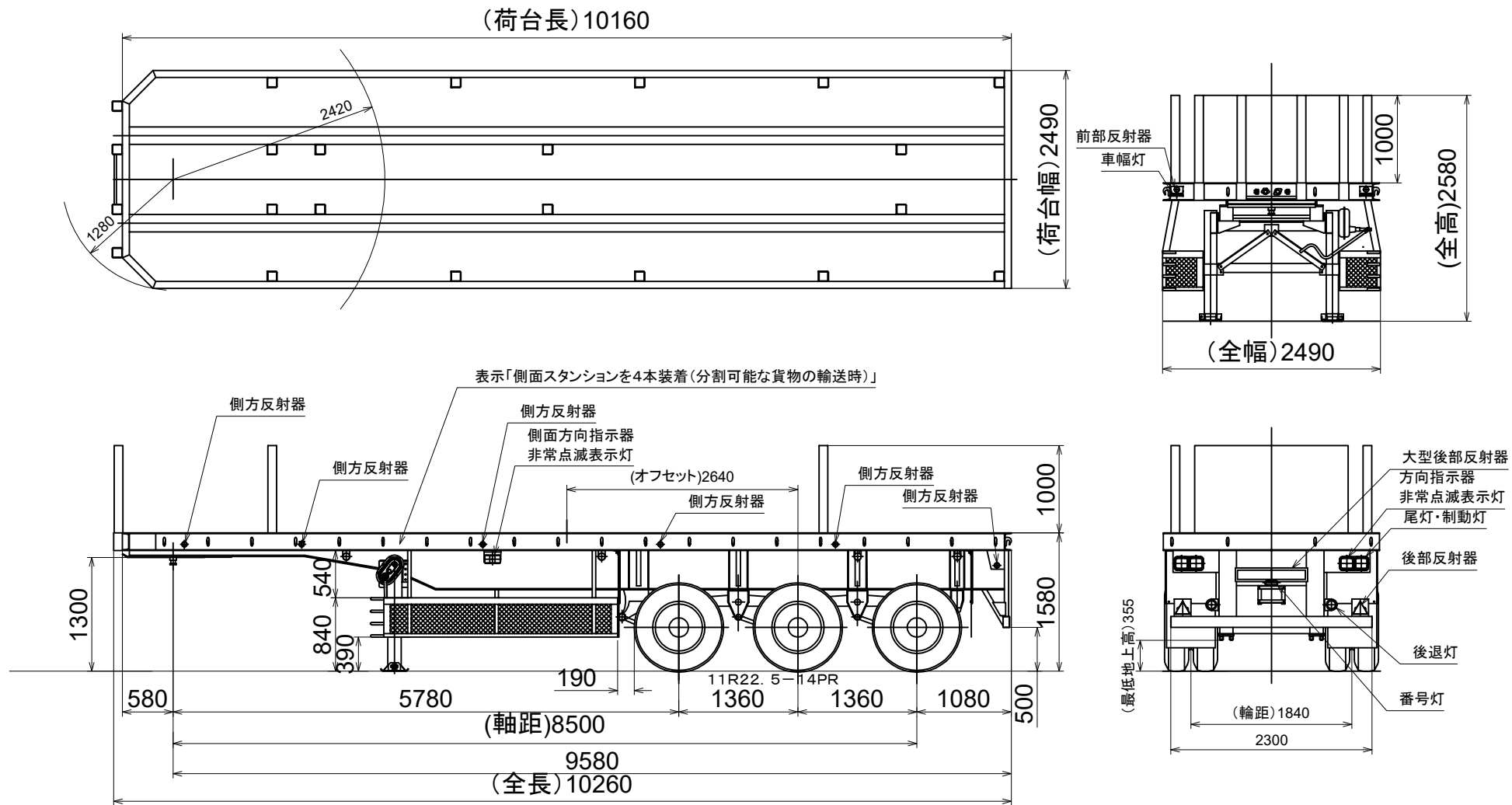
小川建機 YTF45S01 型セミトレーラ外観四面図
